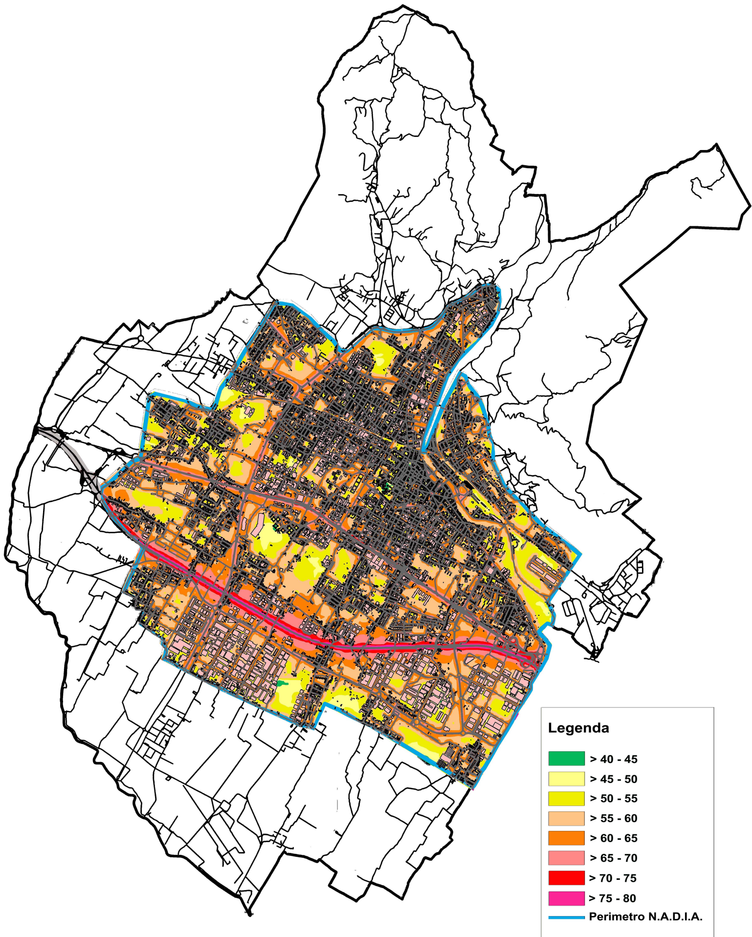
Curve isofone relative al rumore stradale ed all'indicatore Lden
